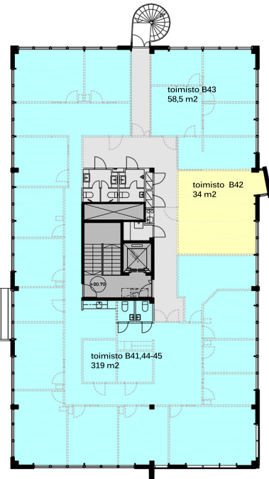
4. KERROS OSA B HUONEISTOALA 473 m 2
