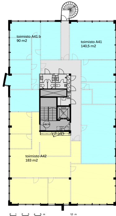
4. KERROS OSA A HUONEISTOALA 473 m 2
